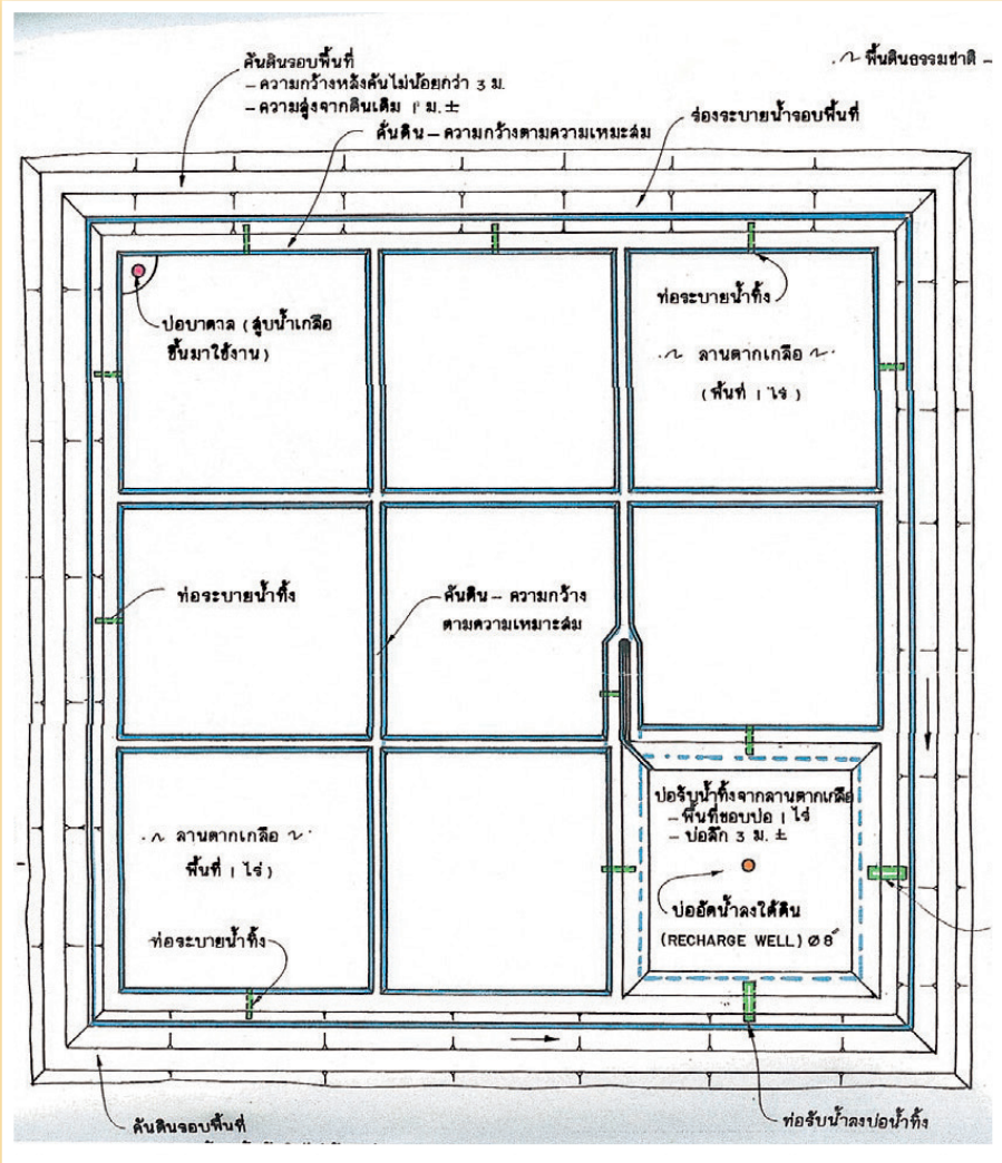
แผนภาพพระราชทานระบบการทำนาเกลือสินเธาว์ตามแนวพระราชดำริ
